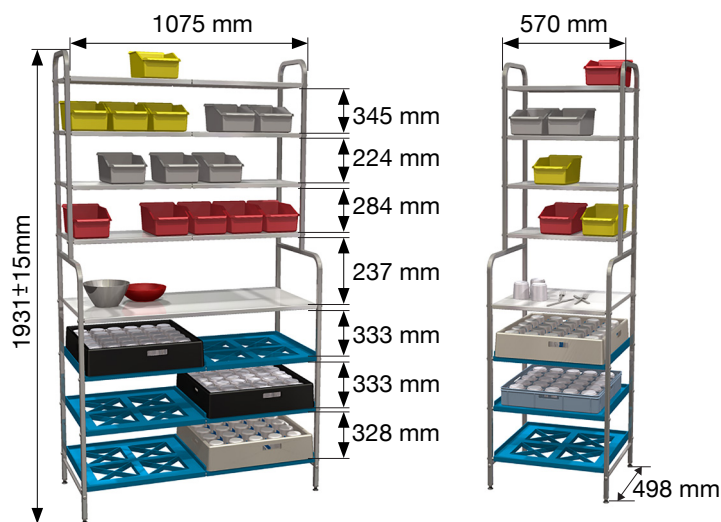
Art.nr. 913 6 korgplatser
