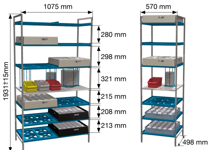
Art.nr. 911 12 korgplatser
