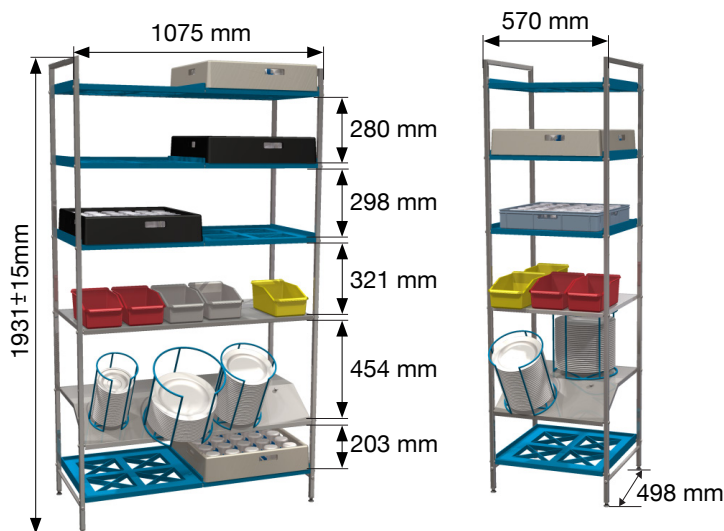
Art.nr. 907 8 korgplatser
