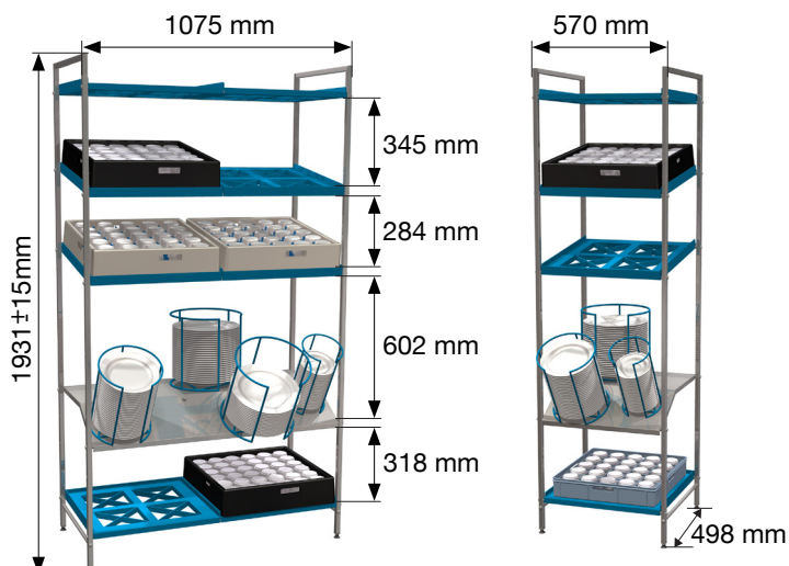
Art.nr. 903 8 korgplatser
