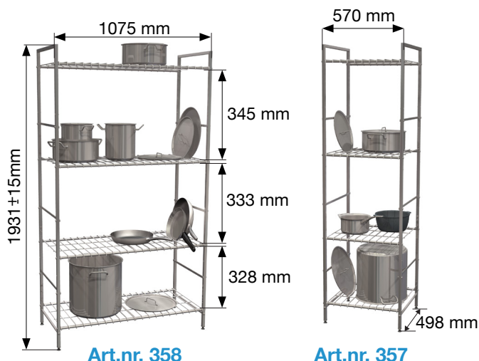
Art.nr. 358
