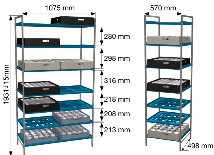
Art.nr. 909 14 korgplatser
