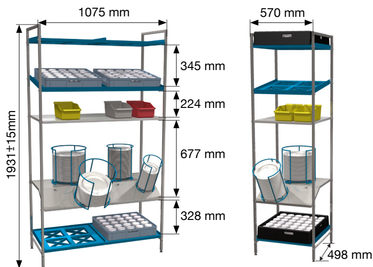
Art.nr. 905 6 korgplatser
