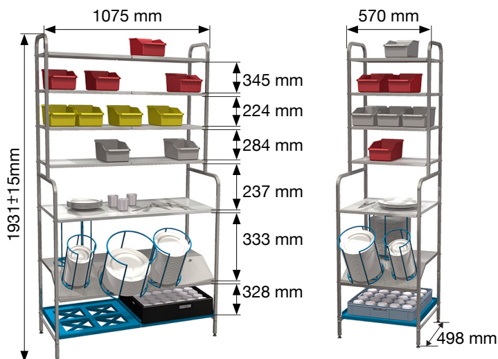
Art.nr. 915 2 korgplatser
