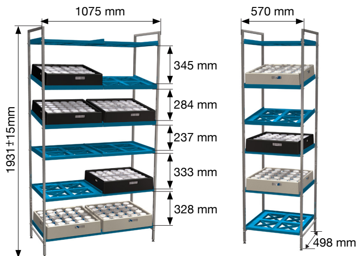
Art.nr. 901 12 korgplatser
